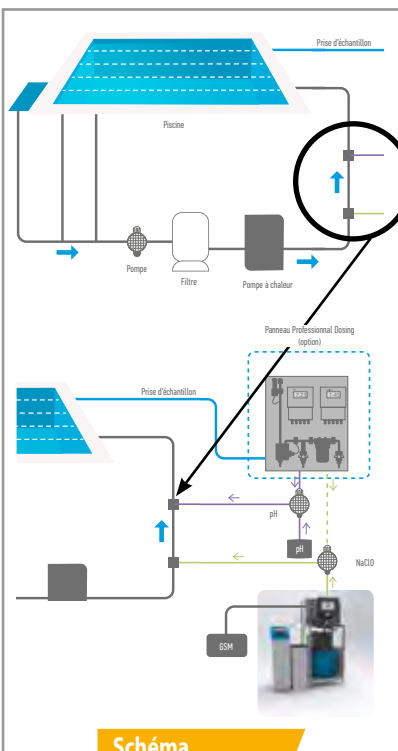
Schéma d'installation Elyseo
